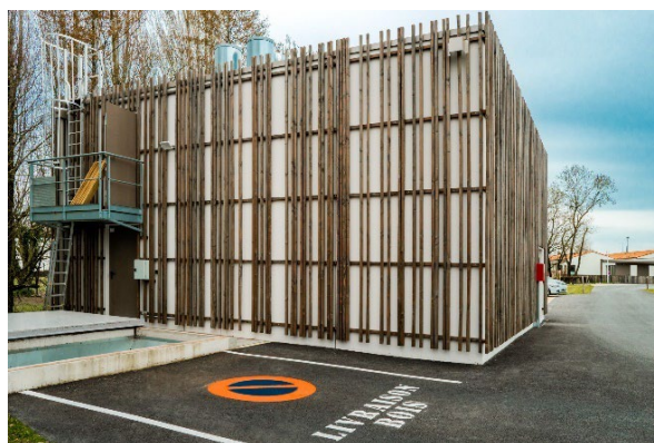
La chaufferie bois de Treize-Septiers alimente 4 bâtiments avec un réseau de chaleur ©SYDEV-Pierre Ollier
